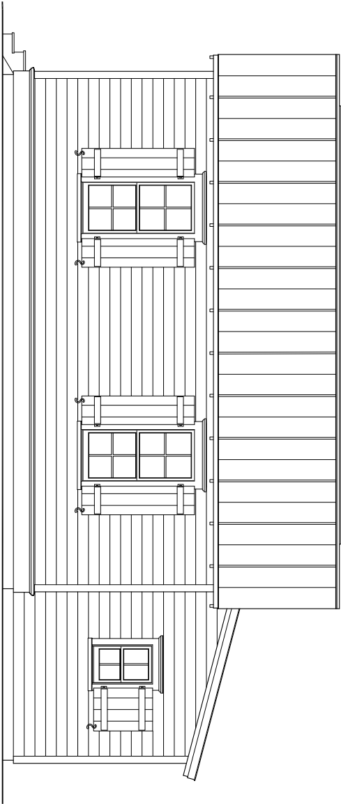
C RIGHT ELEVATION
